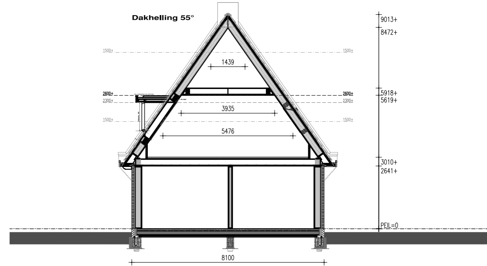
PRINCIPE DOORSNEDE
