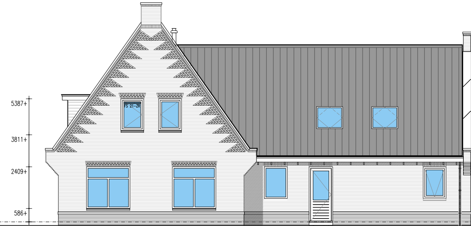
RECHTER ZIJGEVEL
